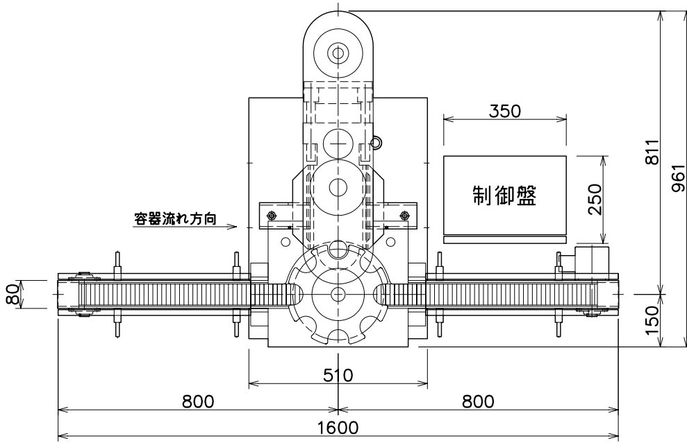
トップチェーンPOM 幅60 ピッチ12.7mm ボトルインデックスPCD260mm
