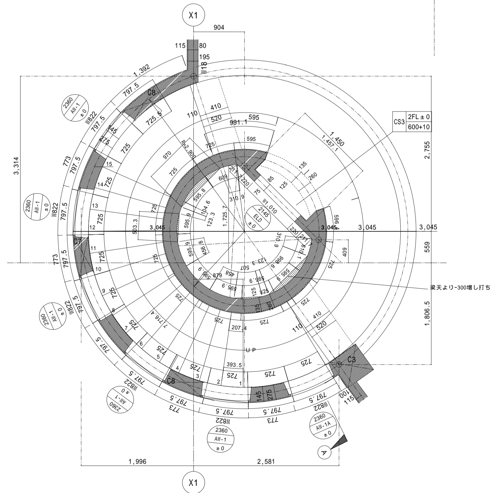
1 F 階段躯体図 S=1/40
