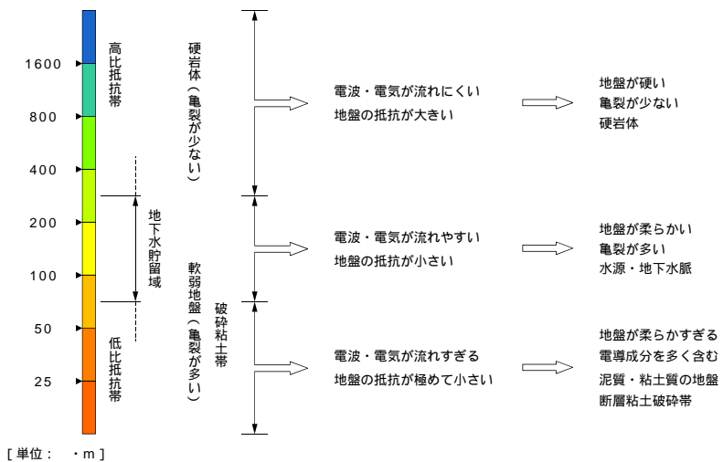
比抵抗値が示す地盤・地下水特性
